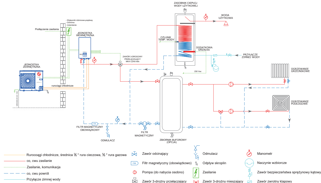
SCHEMAT HYDRAULICZNY
