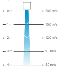
PRĘDKOŚĆ PRZEPŁYWU POWIETRZA
