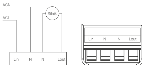
Schemat podłączenia
